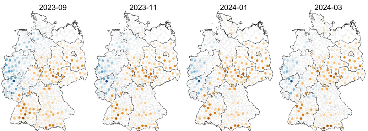
Abb. 3: Saisonale Vorhersagen (2023-Sep bis 2024-Mär) ; Mittel der Anomalien des Bodenspeichers, ParFlow/CLM Simulationen (initialisiert: 2023-09-01) mit ECMWF SEAS Antrieb (50 Ensemble Member). Punkte: NUTS-3 Verwaltungsebene; Punktgröße: Proportional der Anzahl der Member mit identischem Vorzeichen (positive oder negative Anomalie).
