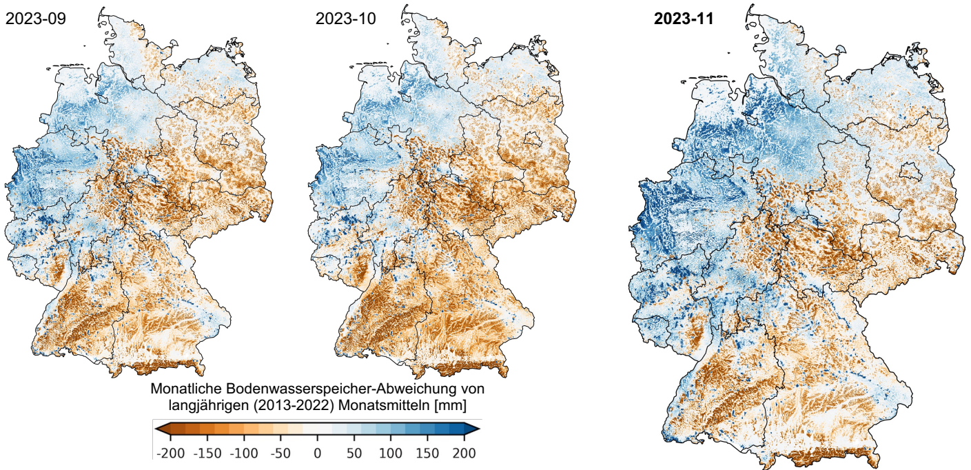
Abb. 1: Monatliche Gesamtspeicherabweichung der vergangenen Jahreszeit mit Bezug auf die langfristigen Monatsmittel von 2013 bis 2022 in mm Wassersäule für die oberen 60m des Bodenspeichers. Daten: Hindcasts von ParFlow/CLM Simulationen, angetrieben mit ECMWF HRES.
