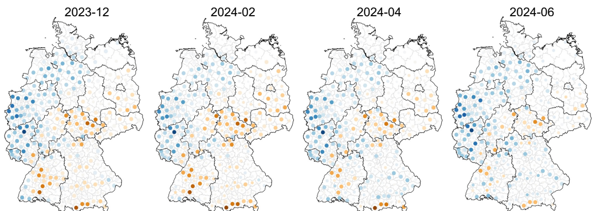
Abb. 3: Saisonale Vorhersagen (2023-Dez bis 2024-Juni) ; Mittel der Anomalien des Bodenspeichers, ParFlow/CLM Simulationen (initialisiert: 2023-12-01) mit ECMWF SEAS Antrieb (50 Ensemble Member). Punkte: NUTS-3 Verwaltungsebene; Punktgröße: Proportional der Anzahl der Member mit identischem Vorzeichen (positive oder negative Anomalie).
